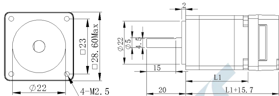
图 6.1 IDH28 系列一体机外观示意图
