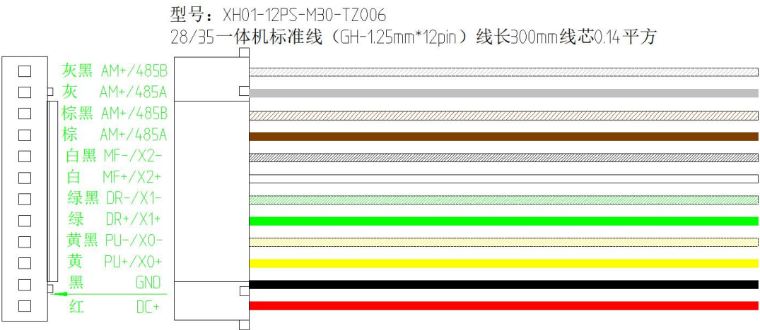
图 6.2 IDH28 系列配线示意图
