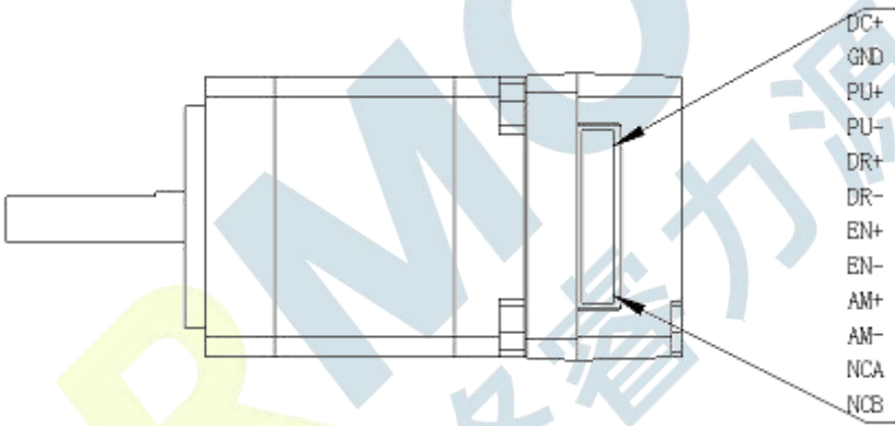
图 3.1 ISS28 接口示意图
