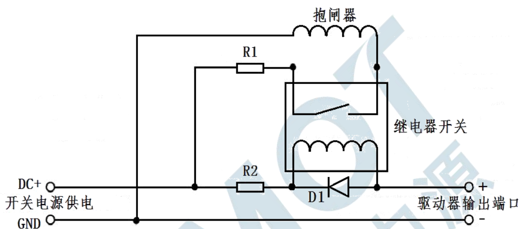
图 3.6 刹车电机抱闸器接线示意图
