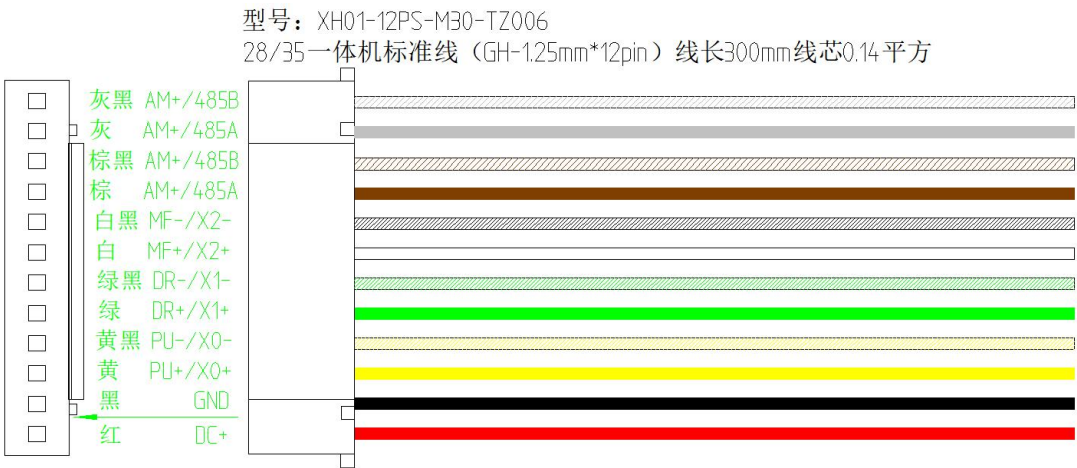
图 6.2 ISS28 系列配线示意图
