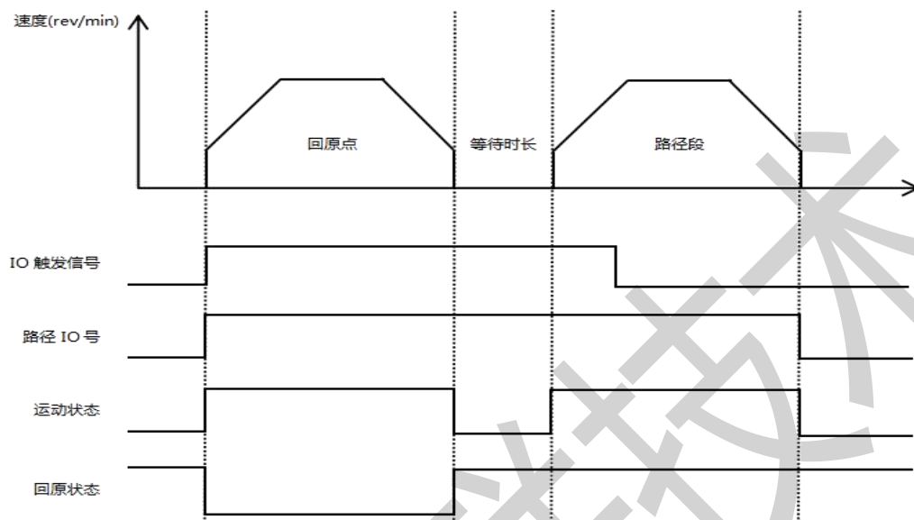
图 5.5 回原点+IO 触发+路径 IO 模式运行示意图
