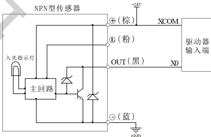
图 3.4 NPN 型传感器接线示意图
